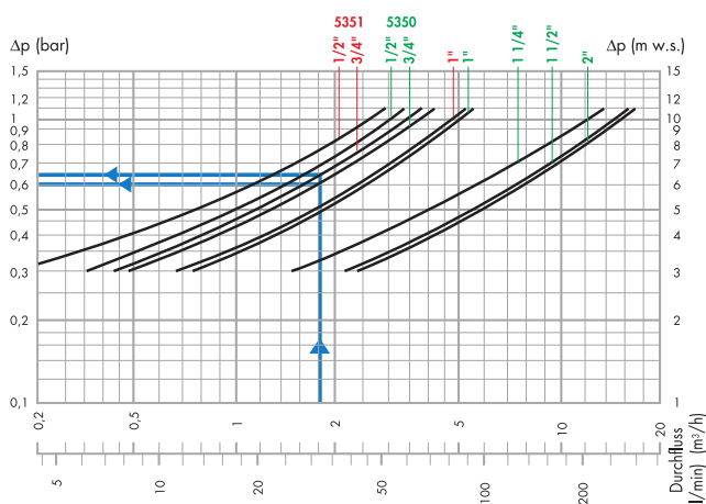
Abbildung 2 (Druckverlust)
