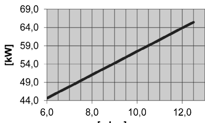
Abb. 25: Leistungsdiagramm RE 1.60 H
