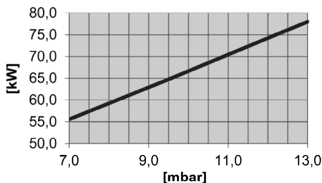
Abb. 26: Leistungsdiagramm RE 1.70 H
